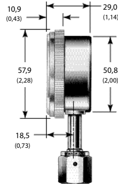
Крепление снизу
