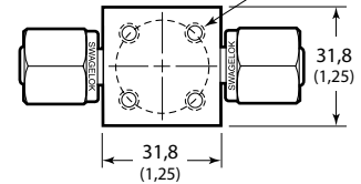
ALD6, вид снизу
