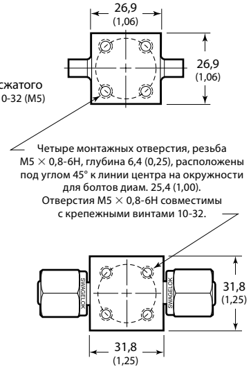
ALD6, вид снизу
