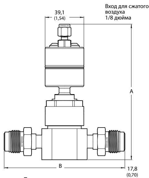
Торцевые соединения в виде поворотного фитинга VCR с наружной резьбой
