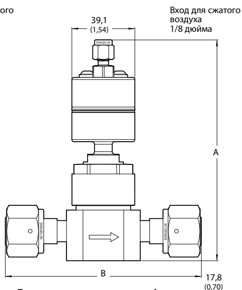
Торцевые соединения в виде фитинга VCR с внутренней резьбой
